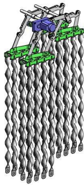
1,2 Wärmetauscher- -Reinigung
