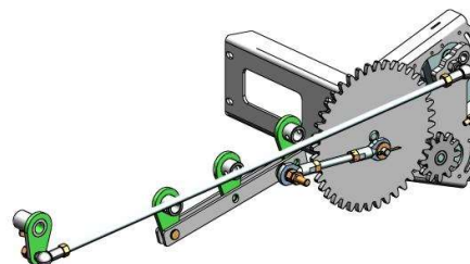
4,4 Antrieb
