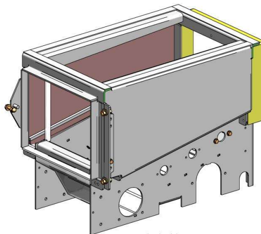
4,1 Koerper
