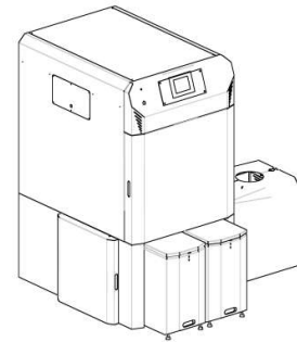
5,1 Verkleidung Kessel
