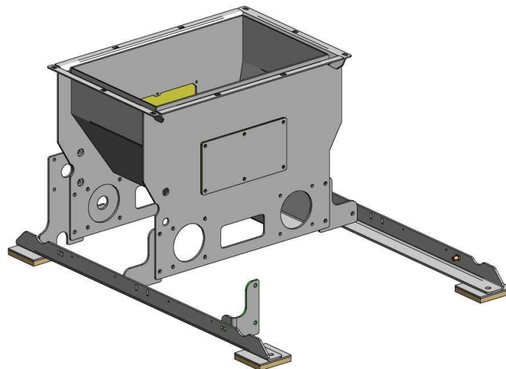
8-1 Unterteil Koerper
