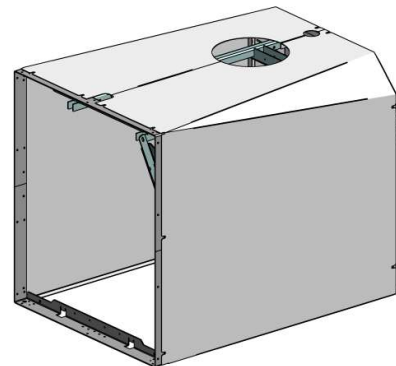
5,5 Verkleidung Einschub
